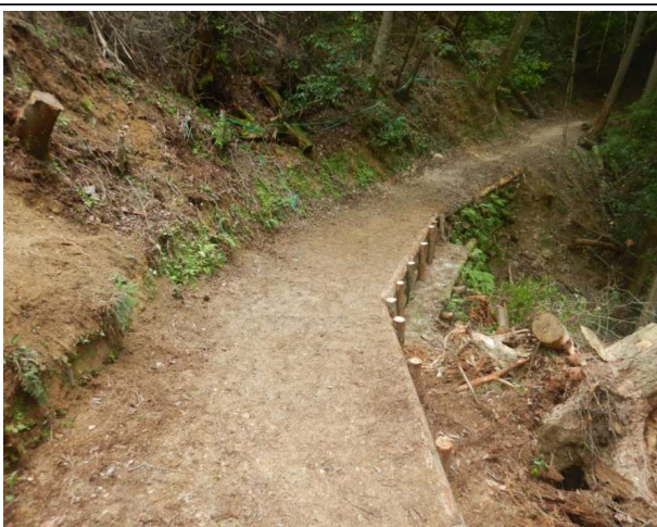
熊野参詣道小辺路(倒木及び崩土撤去修繕)
